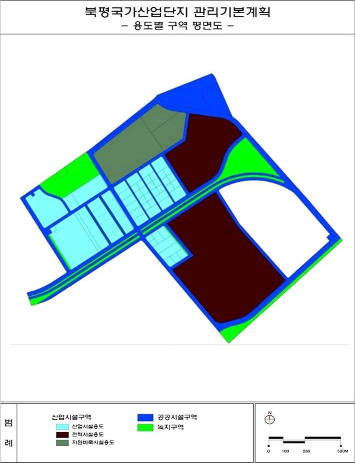
(별첨#1) 북평국가산업단지 용도별 구역 평면도
